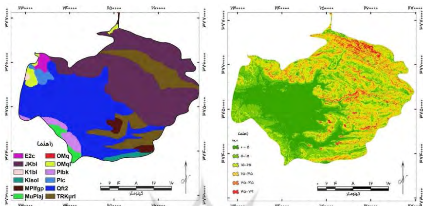
شکل (۲) نقشه شیب منطقه مورد مطالعه شکل (۳) نقشه لیتولوژی منطقه مورد مطالعه
