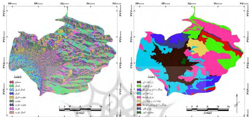
شکل (۵) نقشه جهت شیپ منطقه مورد مطالعه
