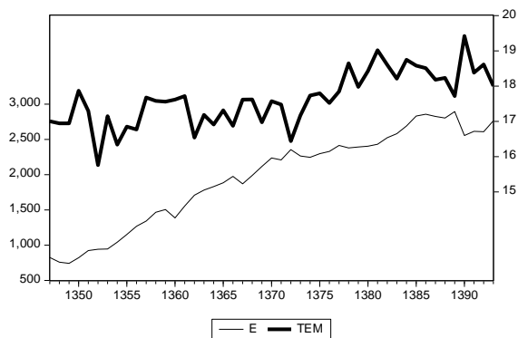
نمودار ۵. رابطه بین دما و مصرف سرانه برق
