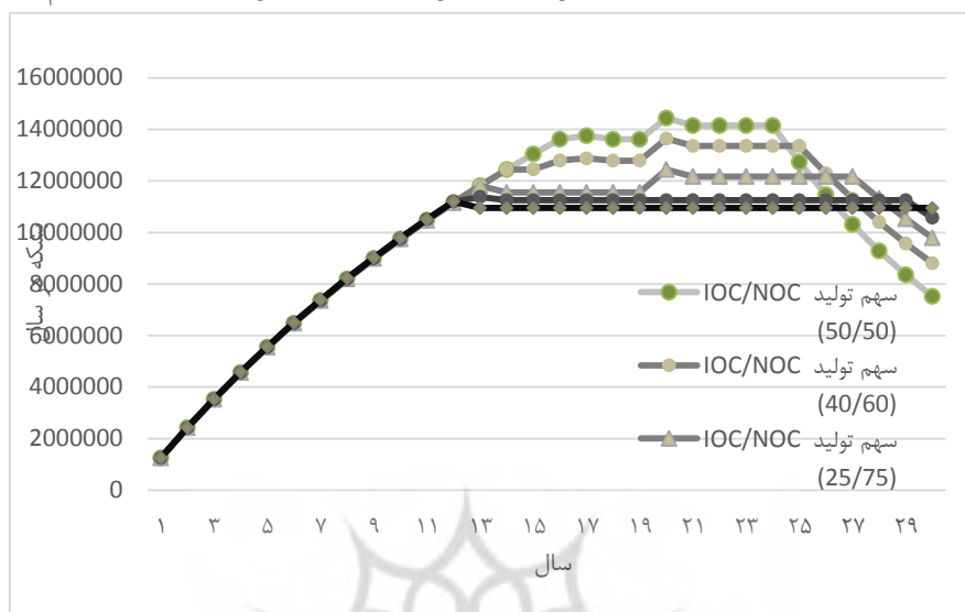
نمودار ۱: روند تخمینی تولید از مخزن در رژیم‌های مالی مختلف قراردادی منبع: محاسبات پژوهش
