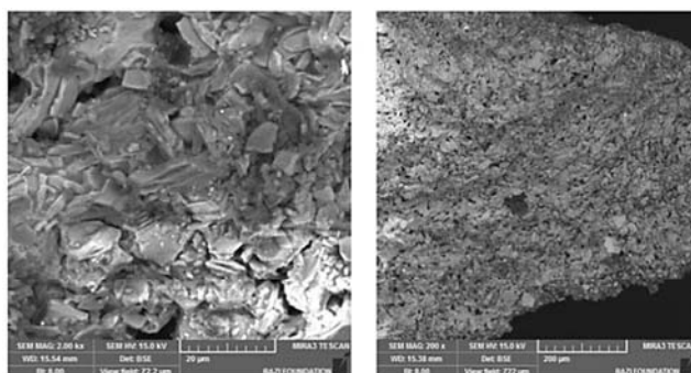
شکل ۸: تصاویر SEM نمونه شماره ۲ راست بزرگنمایی ۲۰۰ برابر - چپ بزرگنمایی ۲۰۰۰ برابر Fig 8: SEM images of sample No. 2 Right: magnified 200x, Left: magnification 2000x
