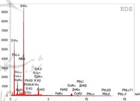
شکل ۱۷: طیف EDX نمونه شماره ۷
