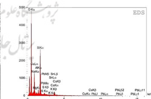
شکل ۵: طیف EDX نمونه شماره ۱ Fig 5: EDX spectrum of sample No. 1
