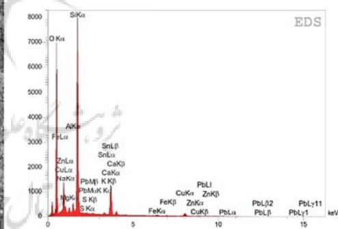
شکل ۲۵: طیف EDX
