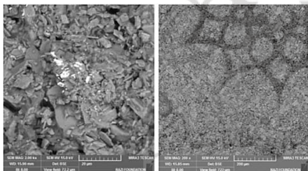
شکل ۱۴: تصاویر SEM نمونه شماره ۵
