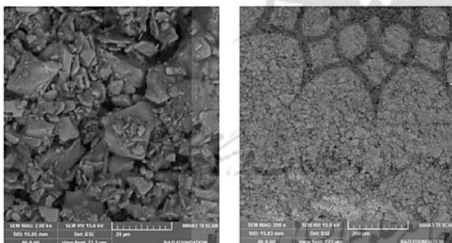
شکل ۱۰: تصاویر SEM نمونه شماره ۳ راست بزرگنمایی ۲۰۰ برابر - چپ بزرگنمایی ۲۰۰۰ برابر Fig 10: SEM images of sample No. 3 Right: magnified 200x, Left: magnification 2000x
