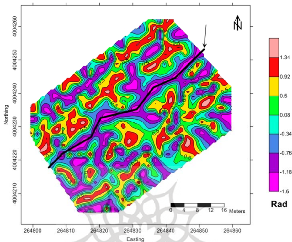
شکل ۵: نقشه اعمال فیلتر زاویه تمایل روی پی‌هنجاری گرانی محدوده مورد مطالعه Fig. 5: Tilt angle map of gravity data covering study area, Tepe Hissar
