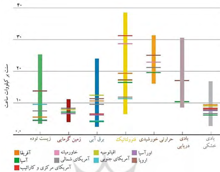
شکل (۱): هزینه تمام شده تولید برق فناوری های تجدیدپذیر منبع: آژانس بین المللی انرژی های تجدیدپذیر، ۲۰۱۴
