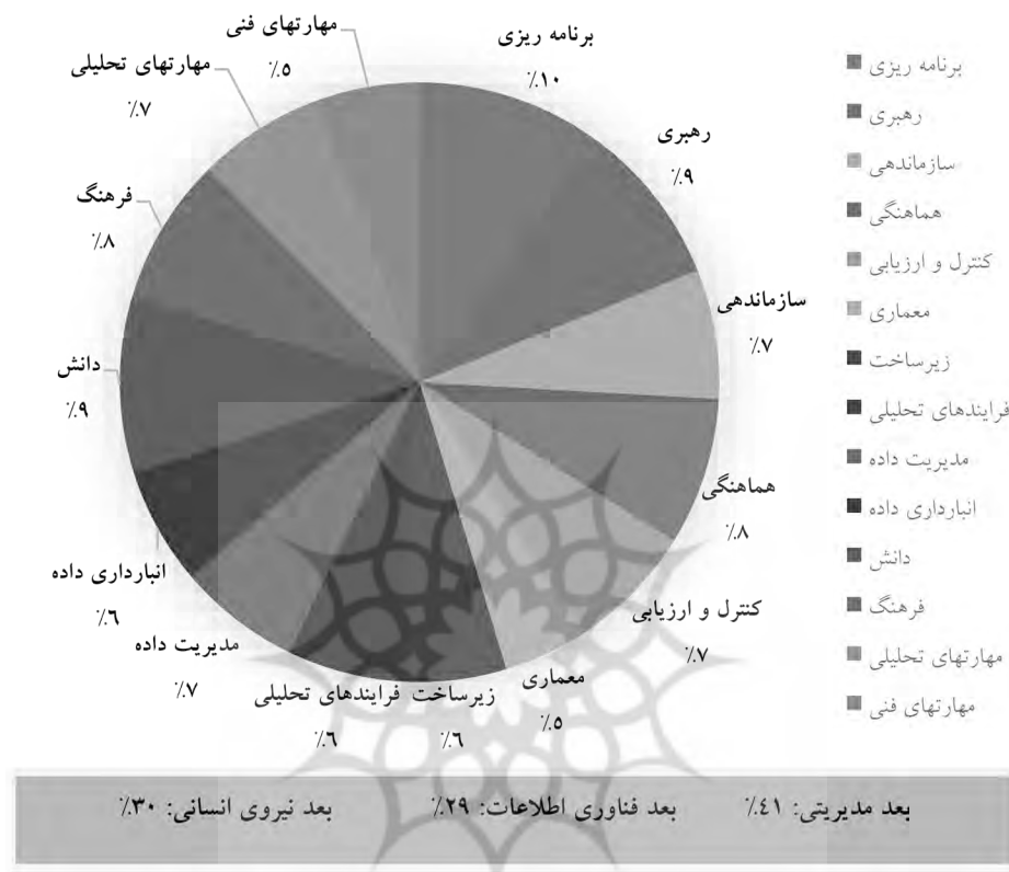
نمودار ۱) ابعاد و ضرایب آن‌ها در مدل ترکیبی پژوهش
