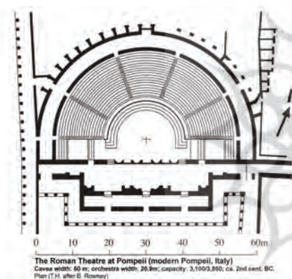
تصویر ۴- ب) پلان، تئاتر پُمپئی، نمونه تئاتر رومی (سایت www.whitman.edu )
