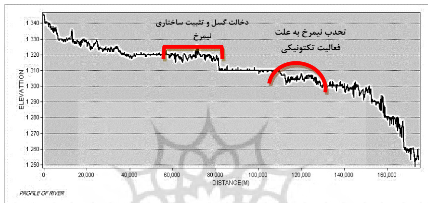
شکل ۱۳: نیمرخ طولی رودخانه قره‌سو در سال ۱۳۹۳
