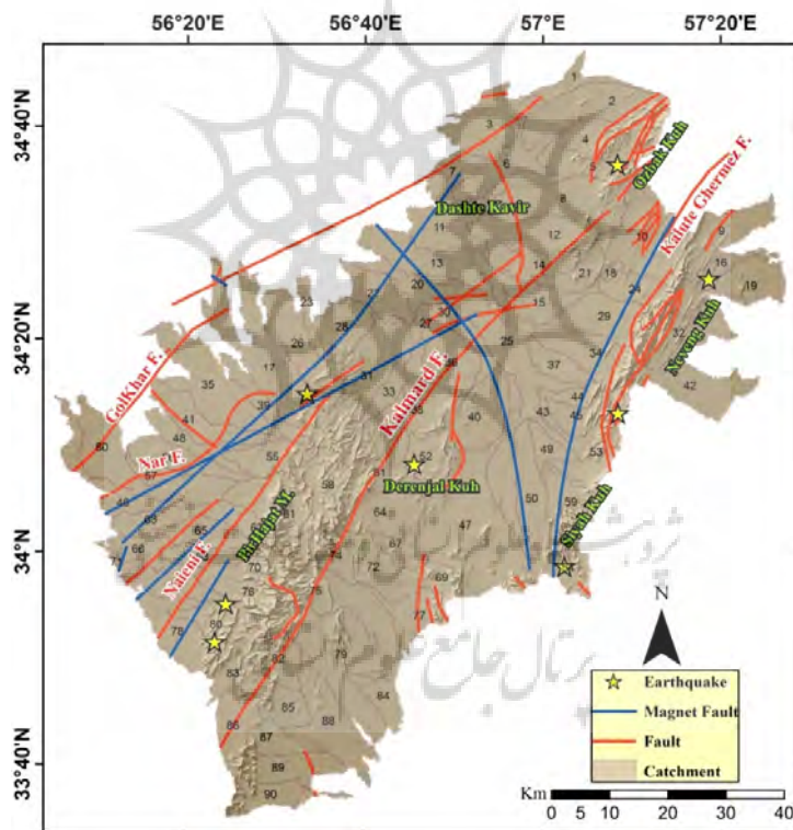
شکل ۱: نقشه پراکنندگی زلزله‌های وقوعی در محدوده‌ی مورد مطالعه
