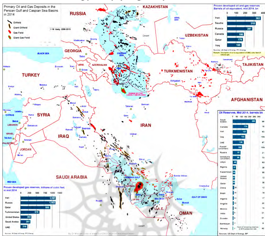
شکل شماره ۲- منابع نفت و گاز شمال ایران
