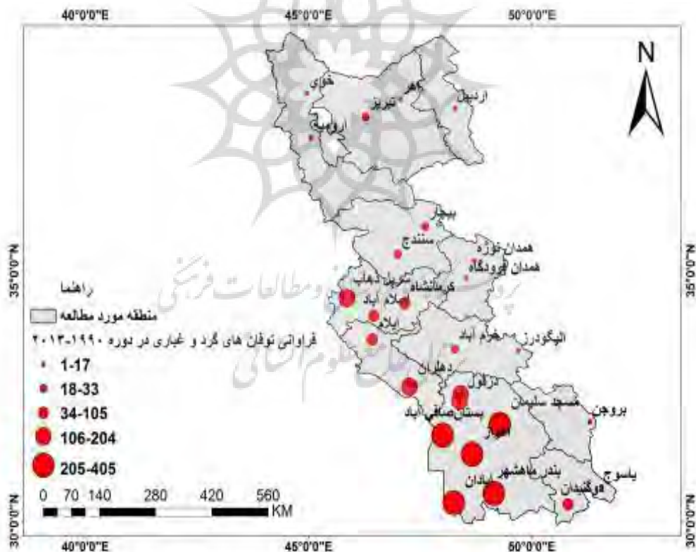
شکل ۲: فراوانی توفان‌های گرد و غباری در نیمه غربی ایران (۱۹۹۰-۲۰۱۳)
