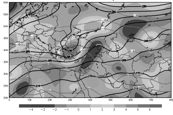
HGT700-VOR700-Temp700
