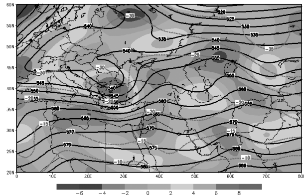
HGT500-VOR500-T500
