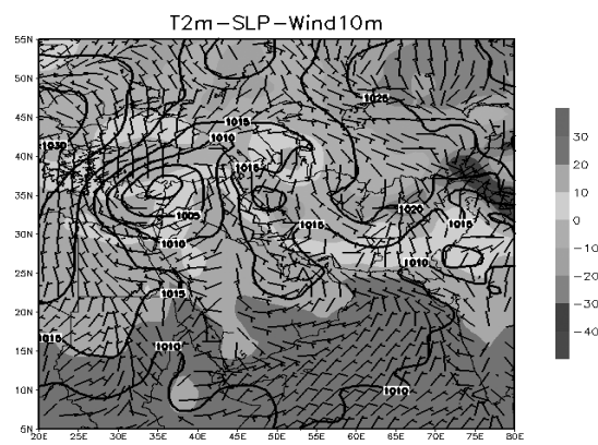
شکل ۲: میدان‌های فشار سطح دریا (خطوط هم‌مقدار بر حسب هکتوپاسکال)، دمای ۲ متری (بخش‌های رنگی شده بر حسب درجه‌ی سلسیوس) و باد ۱۰ متری (بر حسب متر بر ثانیه) برای ساعت ۱۲ گرینویچ روز ۲۹ ژانویه ۲۰۰۸.
