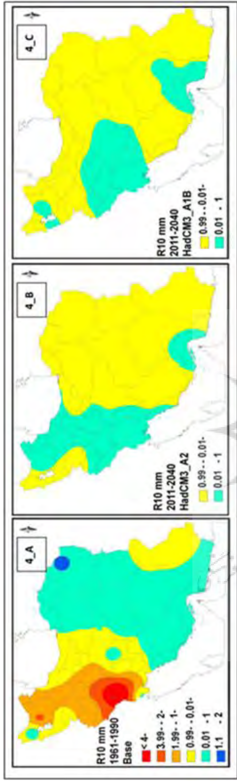
شکل ۴. روند خطی نمایه‌ی روزهای بارش سنگین بر حسب میزان آن بر دهه‌ی طی دوره‌ی پایه (۱۹۶۱-۱۹۹۰) و دوره‌ی آتی (۲۰۱۱-۲۰۴۰).
