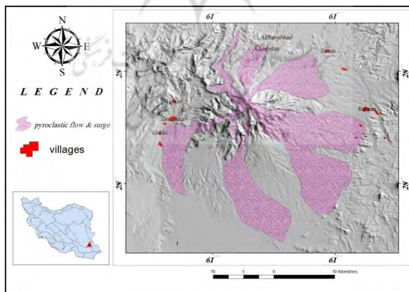
شکل ۱۰ نقشه پهنه‌بندی پیروکلاستیک‌های جریانی در فوران احتمالی آتشفشان تفتان و روستاهای تحت خطر
