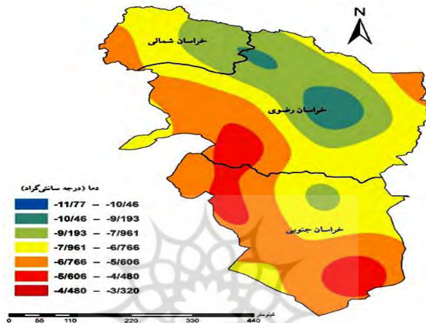
شکل (۵). میانگین بلند مدت دمای حداقل بازه زمانی دسامبر-مارس در منطقه مورد مطالعه (۱۹۵۱-۲۰۱۴)
