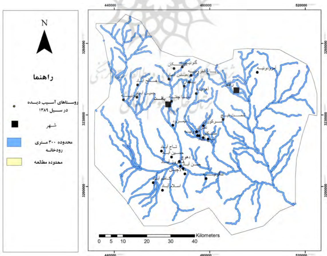
شکل ۲. نقشه حریم ۳۰۰ متری رودخانه‌ها و روستاهای آسیب دیده در اثر سیل تابستان ۱۳۸۹ (منبع: مطالعات نگارندگان)
