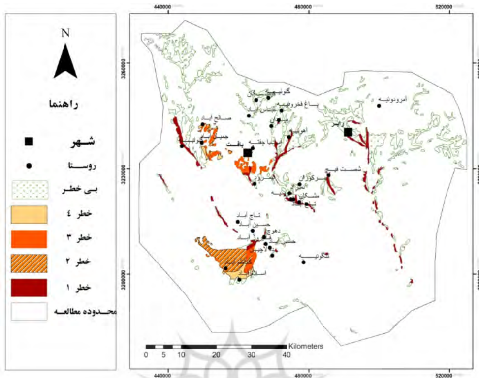
شکل ۳. نقشه کاربری‌های در معرض خطر سیل (منبع: مطالعات نگارندگان)
