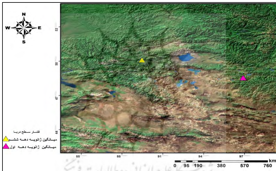
شکل (۴). موقعیت استقرار هسته سامانه پرفشار سیبری در ماه ژانویه در دهه اول و ششم دوره
