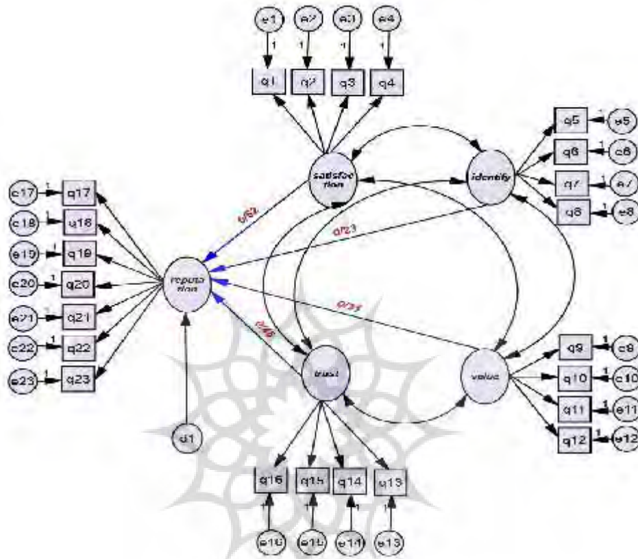
شکل ۱- مدل پژوهش در شرایط تخمین استاندارد
