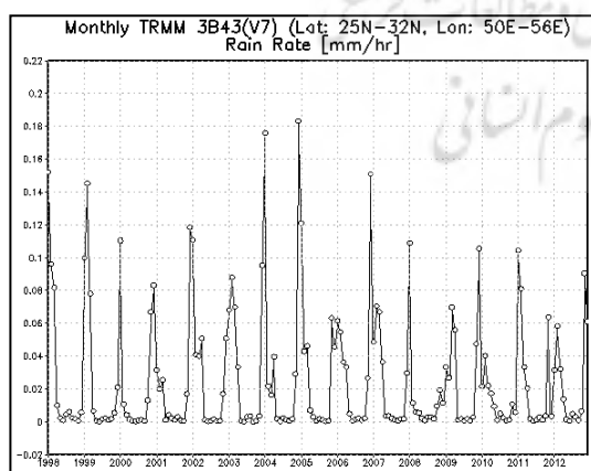
نگاره ۵- روند سالانه شدت بارش میلی‌متر در ساعت
