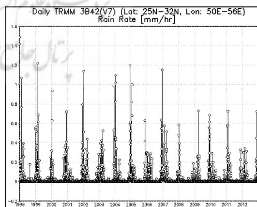
نگاره ۴- روند روزانه شدت بارش میلی‌متر در ساعت
