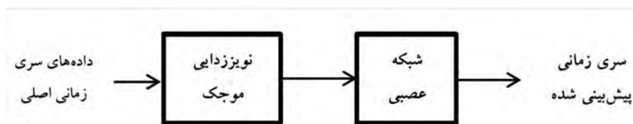
شکل (۲) مدل پیش‌بینی مبتنی بر نويزدایی موجک
