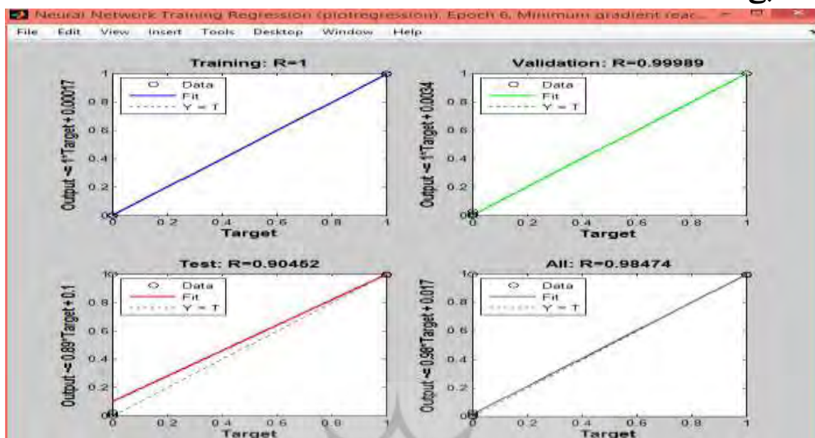
شکل ۳: نمودار رگرسیون
