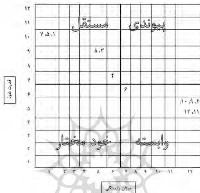
شکل ۲ نمودار MICMAC
