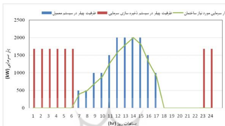
شکل ۲) نمودار بار سرمایه مورد نیاز و تامین شده ساختمان
