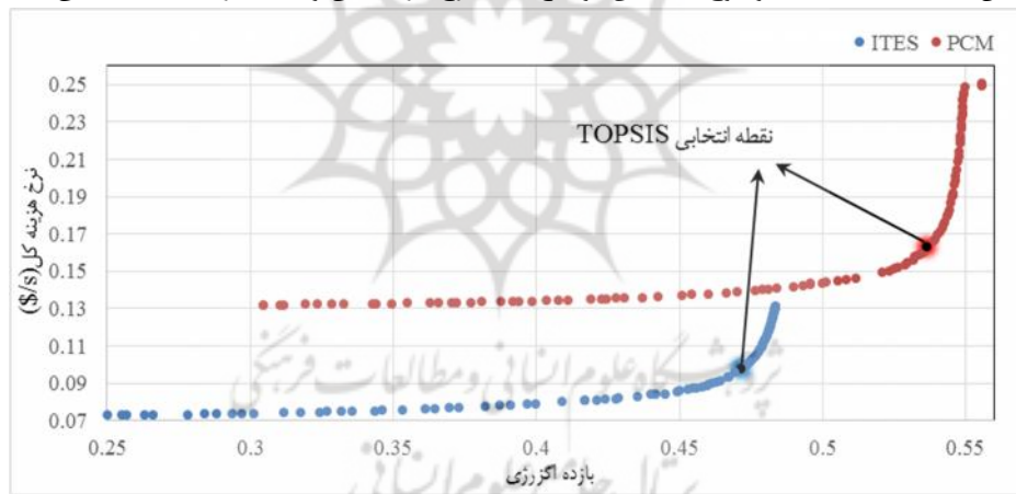
شکل ۴) منحنی بهینه Pareto برای دو سیستم ITES و PCM
