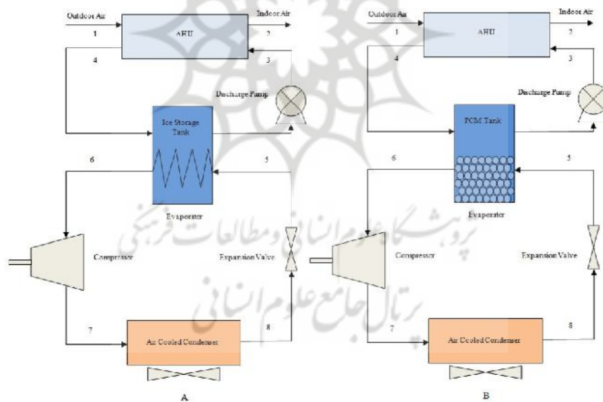
شکل ۱) شماتیک سیستم ذخیره‌ساز سرمایشی ITES (A) و PCM (B)
