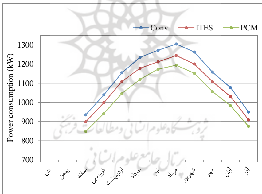
شکل ۵) نمودار مصرف برق سیستم ITES و سیستم PCM و سیستم سرمایشی معمول
