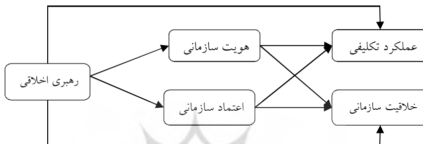
شکل 1 الگوی پیشنهادی پژوهش حاضر، روابط میان متغیرهای پیشاینده، میانجی‌گر و پیامد
