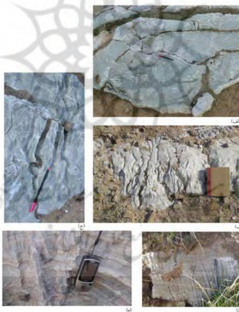
شکل ۲- الف) و ب)، ریل کارن‌ها در رخنمون‌های سطحی گچ (ج)، حرکت موجی رانل‌های گچی، (د) و (ه)، وال کارن‌ها روی دیواره عمودی یک فروچاله ریزشی در لایه‌های گچی سازند گچساران، منطقه آسماری، جنوب شرق مسجد سلیمان، استان خوزستان.
