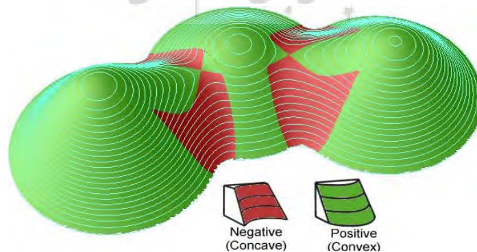
شکل ۳: نمایش شماتیک انحناء سطح و حالت‌های آن (دستورالعمل نرم‌افزار Arc GIS)
