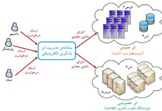
شکل ۴. جگونگی پیاده‌سازی معماری پیشنهادی برای سیستم یادگیری و آموزش الکترونیکی
