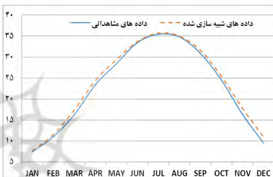
شکل ۸ شبیه‌سازی دمای بیشینه در ایستگاه بیارجمند
