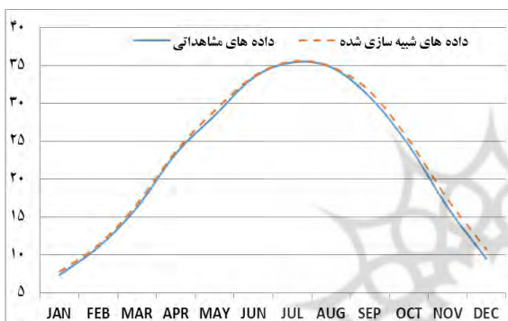
شکل ۹ شبیه‌سازی دمای بیشینه در ایستگاه بیارجمند در
