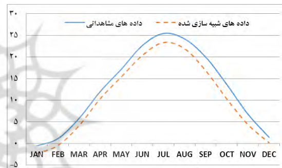
شکل ۳۲ شبیه‌سازی دمای کمینه در ایستگاه سمنان
