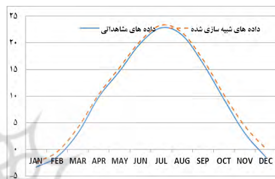
شکل ۶ شبیه‌سازی دمای کمینه در ایستگاه بیارجمند
