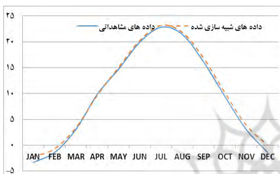
شکل ۵ شبیه‌سازی دمای کمینه در ایستگاه بیارجمند
