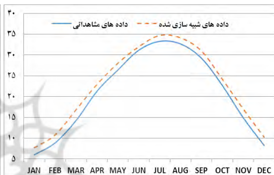
شکل ۱۷ شبیه‌سازی دمای بیشینه در ایستگاه شاهرود
