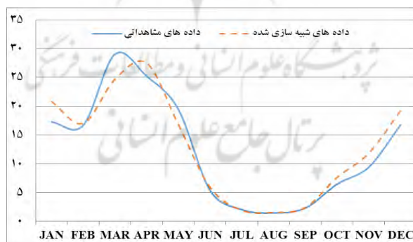
شکل ۱۲ شبیه‌سازی بارش در ایستگاه شاهرود در سناریوی A1B
