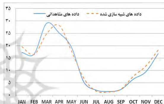
شکل ۱۱ شبیه‌سازی بارش در ایستگاه شاهرود در سناریوی B1
