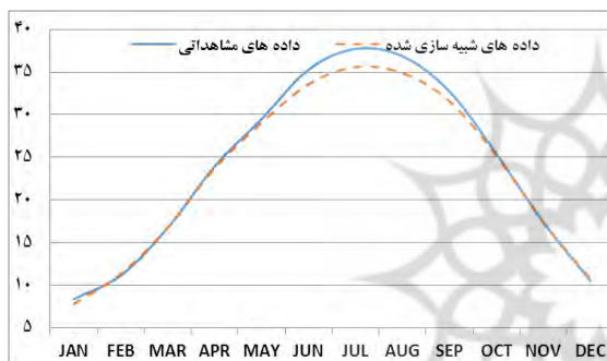
شکل ۳۶ شبیه‌سازی دمای بیشینه در ایستگاه سمنان
