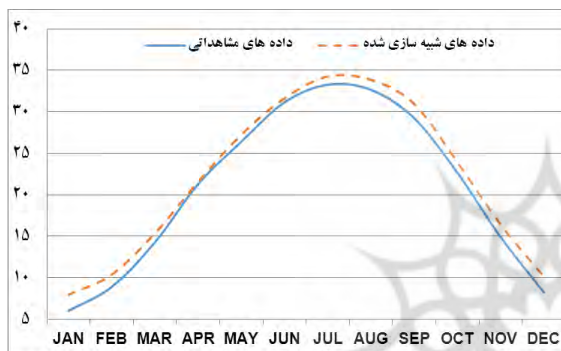
شکل ۱۷ شبیه‌سازی دمای بیشینه در ایستگاه شاهرود
