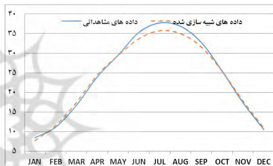
شکل ۳۵ شبیه‌سازی دمای بیشینه در ایستگاه سمنان در
