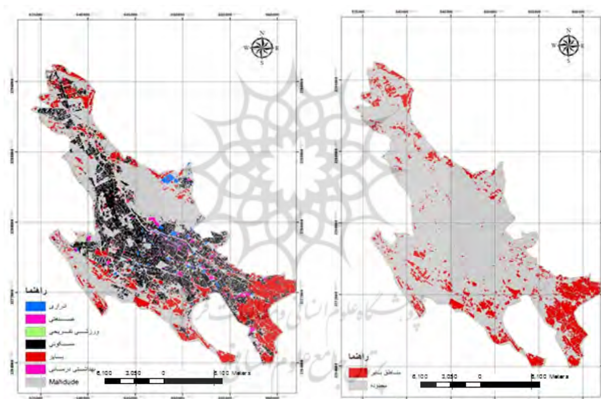
شکل ۲. نقشه کاربری‌های شیراز در سال ۱۳۸۳ (منبع: نگارندگان)
