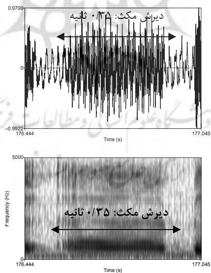
شکل ۳. سیگنال و طیف‌نگاشته مکث پرشده.
