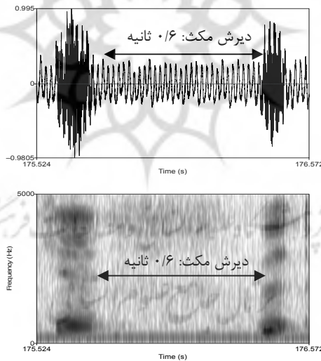
شکل ۱. سیگنال و طیف‌نگاشته مکث تنفسی.
