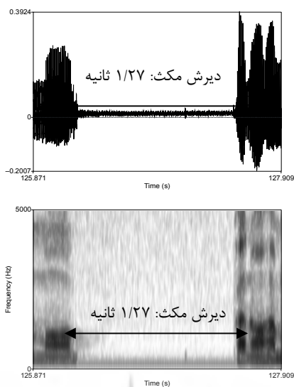
شکل ۲. سیگنال و طیف‌نگاشته مکث ساکت.
