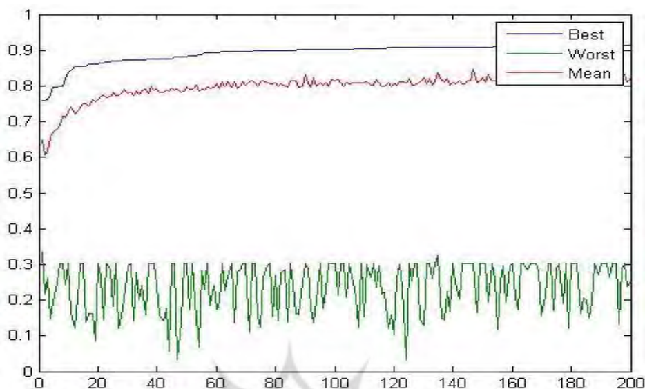
شکل (۷): نمودار همگرایی دیتاست ژاپن
