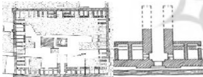
تصویر ۱۲. پلان و مدخل ضلع شرقی دروازه کاخ ساسانی
