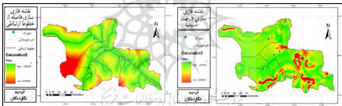
شکل ۷: نقشه فازی سازی فاصله از خطوط ارتباطی و درصد شیب
