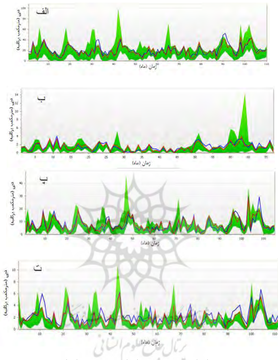
شکل ۲. محدوده باند عدم قطعیت (—)، دبی شبیه‌سازی شده (—) و دبی مشاهده‌ای (—) در دوره واسنجی رواناب ماهانه ایستگاه‌های: الف) کره‌سنگ؛ ب) رزن؛ پ) چالو؛ ت) پنجاب
