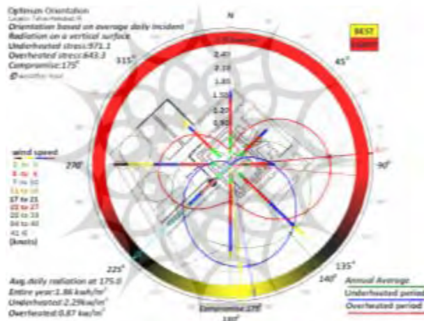
شکل ۶. انطباق پلان سایت در نمودار S.R.W.R (ترکیب بادهای غالب فصل تابستان و زمستان است) (منبع: سلیمانان، ۱۳۹۰: ۷۶)
