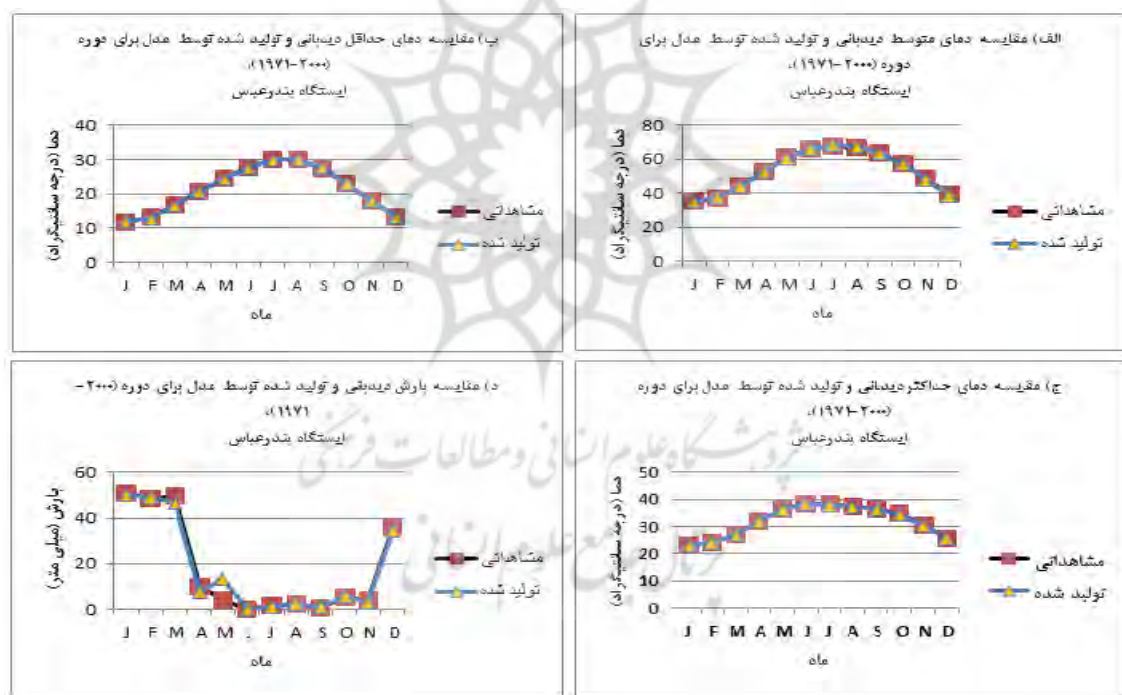
شکل ۳. نتایج حاصل از مقایسه مقادیر مشاهده‌ای و مدل‌سازی شده در ایستگاه بندرعباس برای دوره (۱۹۷۱-۲۰۰۰) با استفاده از مدل LARS-WG برای پارامترهای الف) دمای متوسط؛ ب) دمای حداقل؛ ج) دمای حداکثر؛ د) بارش
