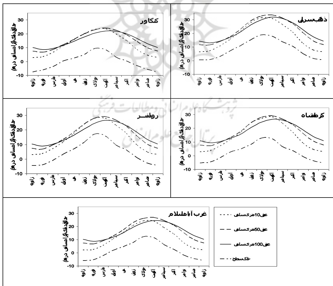
شکل ۳. نمودارهای تغییرات ماهانه‌ی دماهای حداقل خاک در ساعت ۶/۳۰ صبح در ایستگاه‌ها (۲۰۰۶-۱۹۹۳)
