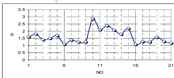
شکل ۷. میزان سینوزیته رودخانه شور جای از محل سد ملاجیغ (قطعه شماره ۲۱) تا محل اتصال آن به رودخانه قرنقو (قطعه شماره ۱). شکل سمت راست. تصویری از یک مسیر ماندری با سینوزیته بالا در مسیر رودخانه شور (شکل سمت چپ).
