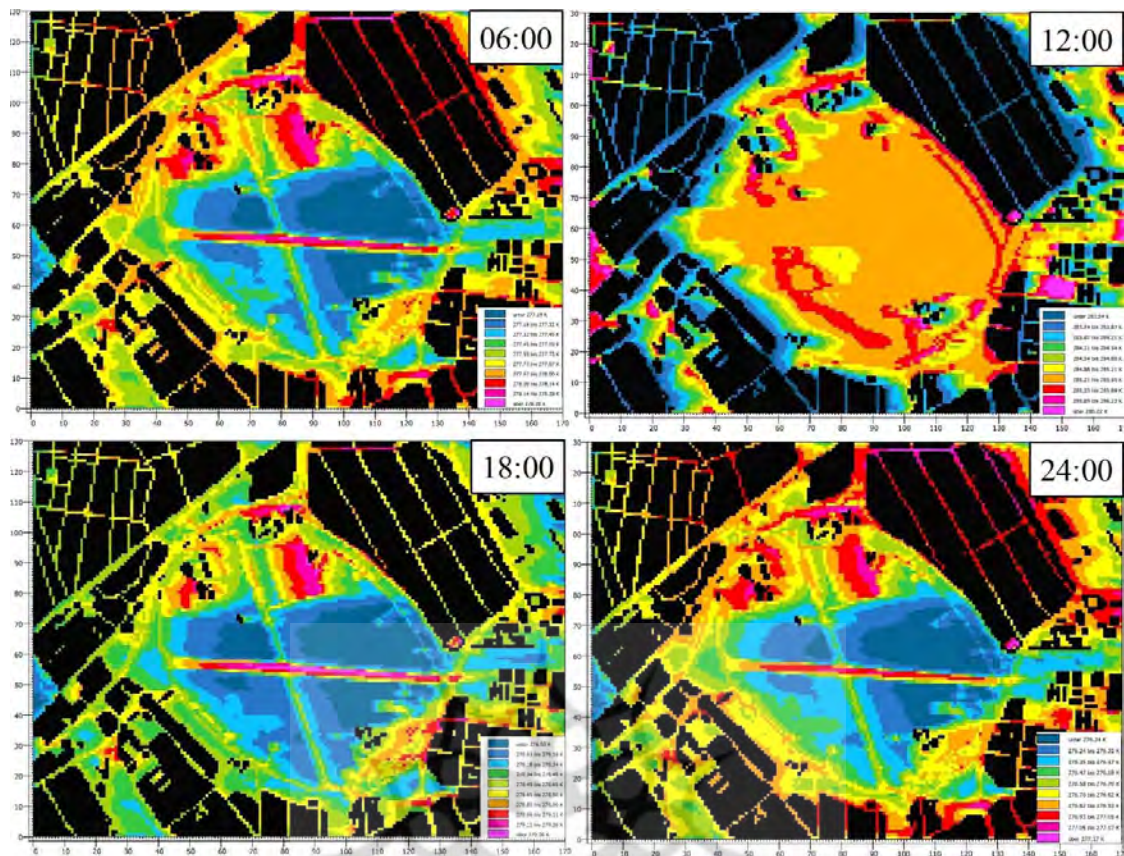
شکل ۳. تغییرات دمای هوا در ساعات‌های ۰۶:۰۰، ۱۲:۰۰، ۱۸:۰۰، و ۲۴:۰۰ روز هفدهم ژانویه ۲۰۱۳
