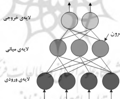
(شکل ۲): شبکه عصبی پرسپترون چندلایه با یک لایه میانی با اندکی تغییر (هورنیک و همکاران، ۱۹۸۹)
