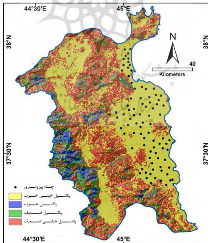
شکل ۱۱. نقشه مناطق دارای پتانسیل آبهای زیرزمین و ارتباط آن با چاه‌های پیزومتری
