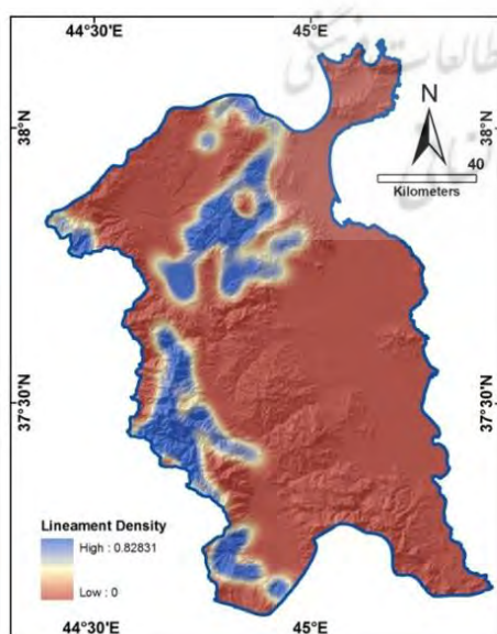
شکل ۷. تراکم خطواره‌ها ( \text{Km}^2/\text{Km}^2 )
