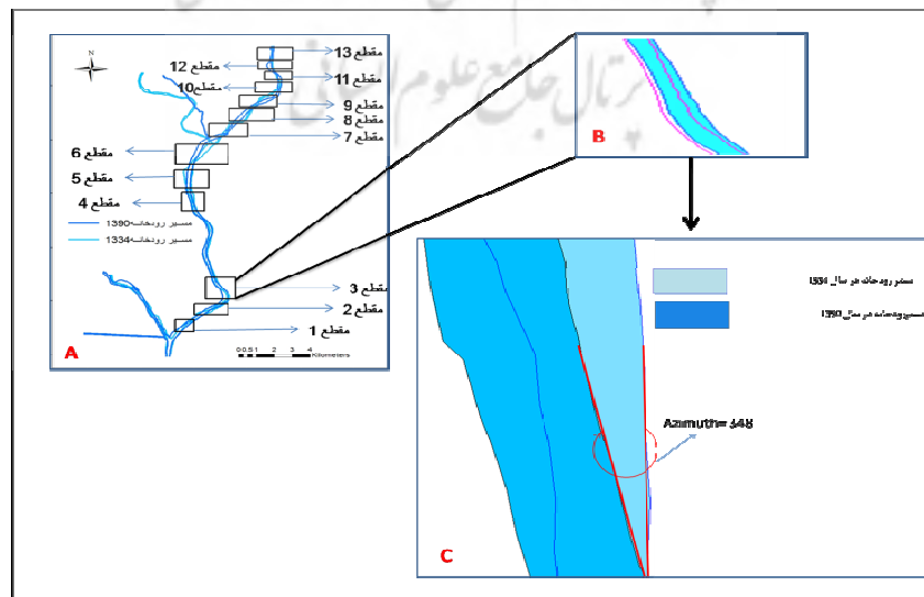
شکل ۴. A. نمای کلی از مقطع بندی رودخانه هیرمند؛ B. مقطع شماره ۳؛ C. چگونگی محاسبه آزیموت (مقطع شماره ۳)
