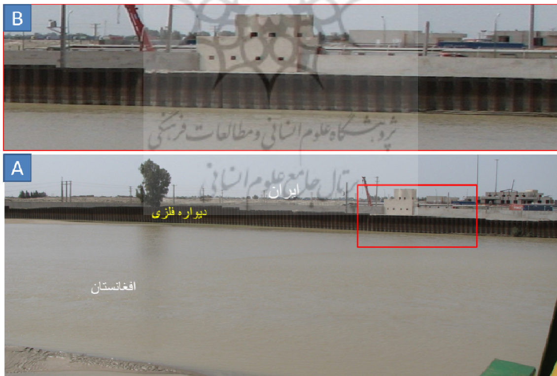
شکل ۸. موانع ساخته شده برای تعدیل فرسایش ساحل غربی هیرمند در محل پل ابریشم و گمرک میلک؛ (A) نمایی از دیواره فلزی ساخته شده؛ (B) نمای نزدیک از مستطیل قرمز در تصویر A معرف دیوار ساحلی و تأسیسات گمرک در ساحل غربی
