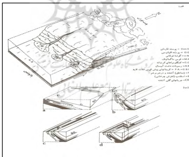
شکل ۳. چین‌های تراستی و تراست تکتونیک و مدل فرورانش در منطقه‌ی بینالود
