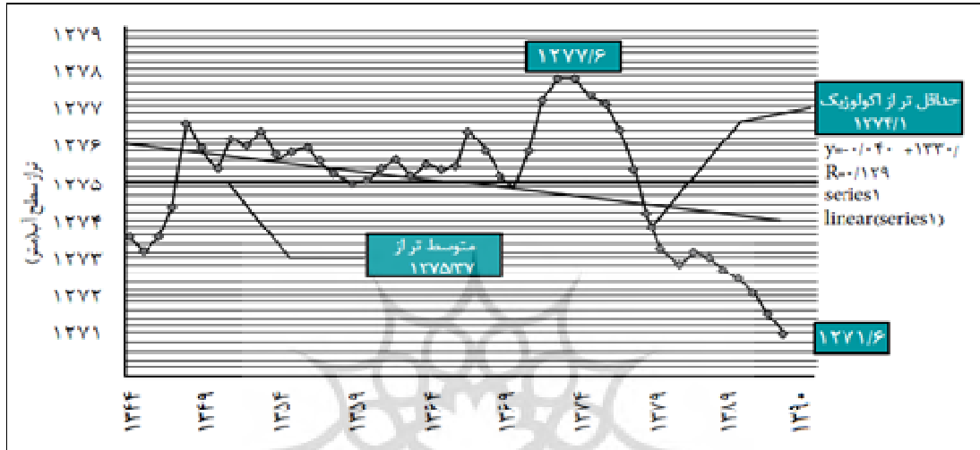
شکل ۵: نمودار تغییرات سطح آب دریاچه ارومیه (۱۳۹۰-۱۳۴۴) ثبت شده به وسیله ماهواره TOPEX/ Jason
