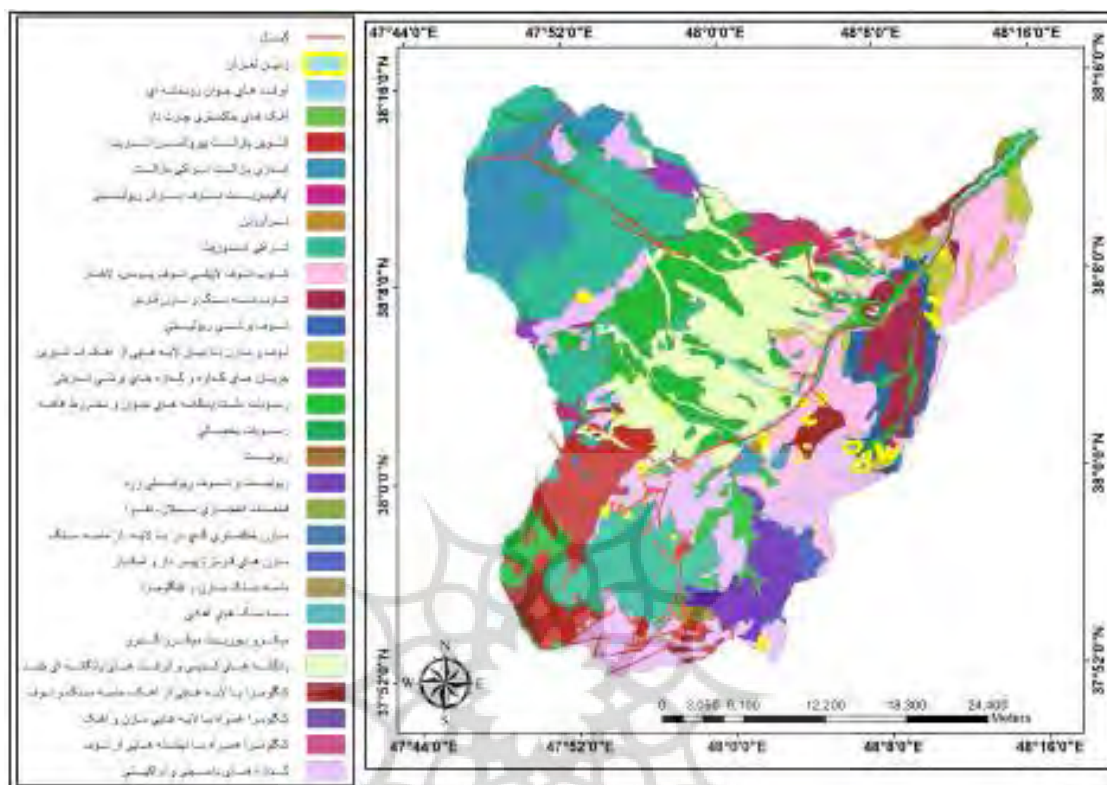
شکل ۴- نقشه زمین‌شناسی به همراه زمین‌لغزش‌های رخ داده در منطقه (منبع: نقشه زمین‌شناسی ۱:۱۰۰۰۰۰ اردبیل، گیوی، مشگین‌شهر و سراب)
