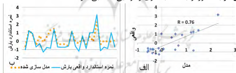
شکل (۱۴). نمودار پراکنش نقطه‌ای و همبستگی (الف) و نمودار خطی (ب) مورد ۲۶ از مقادیر واقعی و مدل‌سازی شده ناهنجاری بارش غرب کشور
