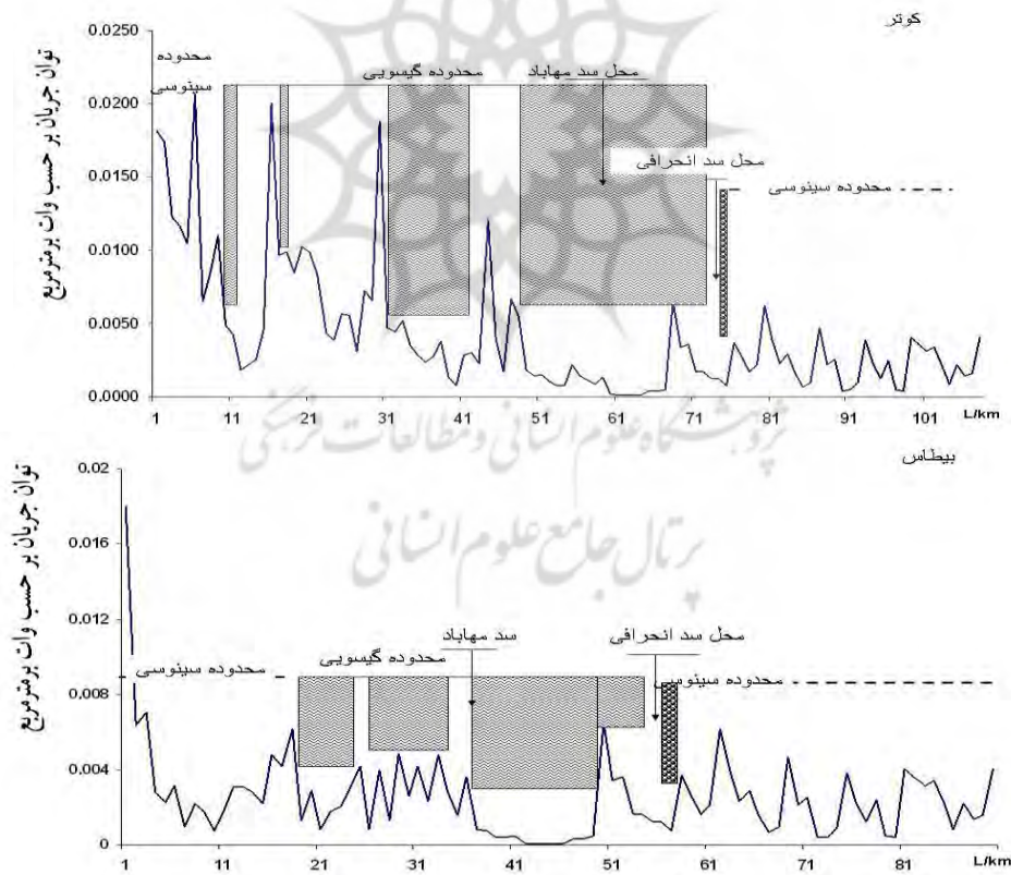
شکل (۷). تغییرات توان جریان و انطباق آن با تغییرات شکل مجرا
