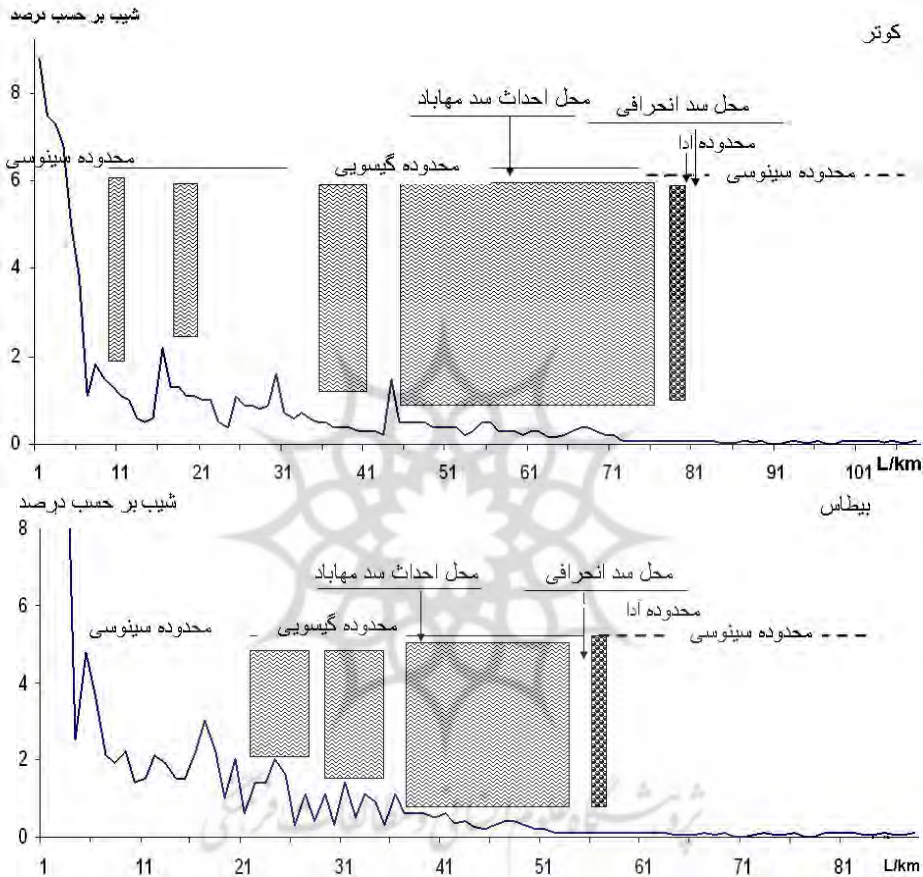
شکل (۵). تغییرات شیب و انطباق آن با تغییرات شکل مجرا
