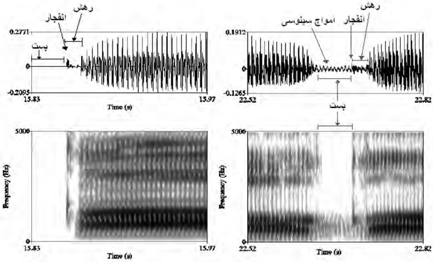
شکل ۲. موج صوتی و طیف نگاشت همخوان ملازی در حالت انسدادی در آغاز واژه (چپ) و جایگاه میان واکه‌ای (راست). زنجیره‌های نشان داده شده عبارتند از /aqa/ از کلمه «آقا» و /ga/ از کلمه «غارت».
