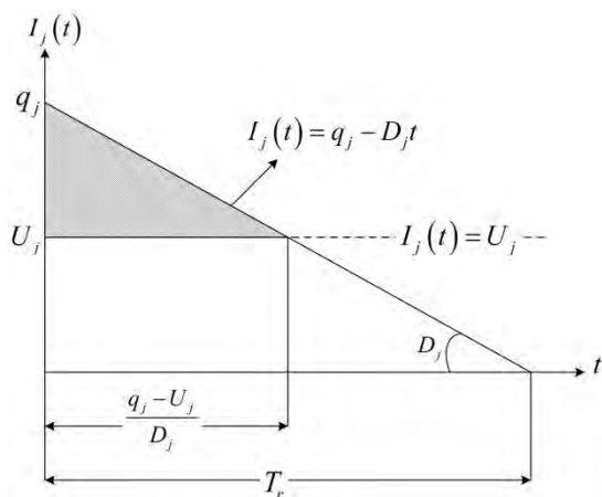
شکل ۲- نمودار موجودی خرده‌فروش لازم برحسب زمان در طول مدت T_r
